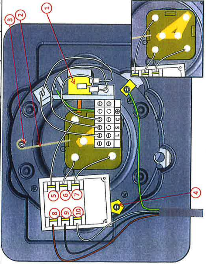
Produit sur socle kit triphasé (On-floor / Three phase product)
