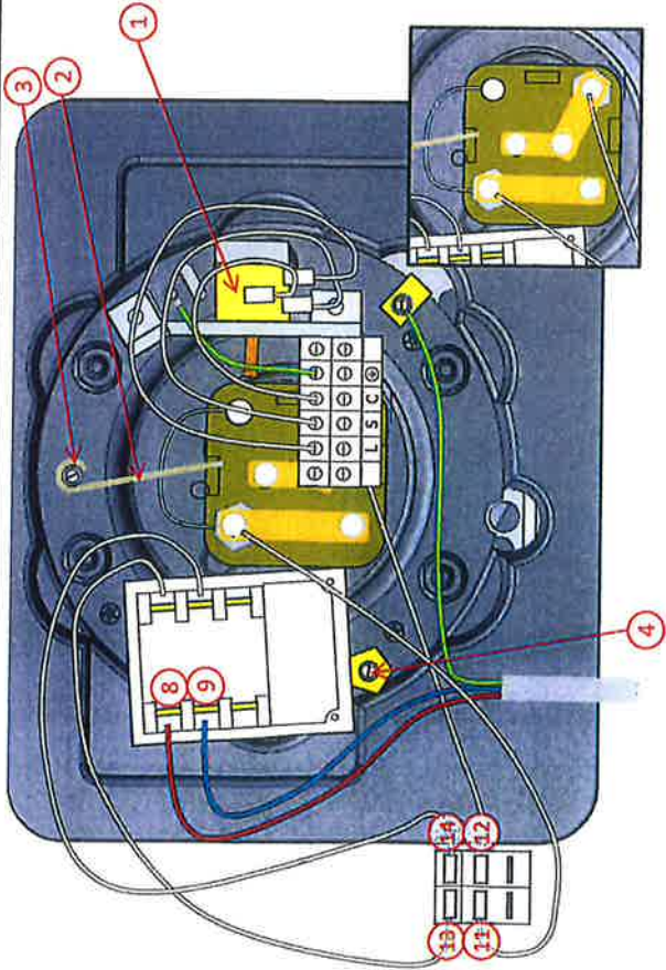
Produit sur socle kit monophasé (On-floor / Single phase product)
